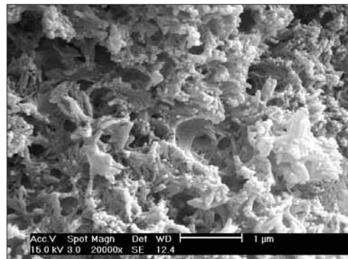
Mikrofotografia cementovej matrice po zmiešaní škárovacej zmesi Keracolor FF s tekutou prísadou Fugolastic. Všímajte si kompaktnejšiu štruktúru spôsobenú obsahom polymérov v škárach.
